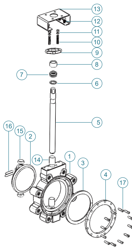
Lug type
